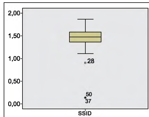
Figura N° 1: Diagrama de caja y bigotes
